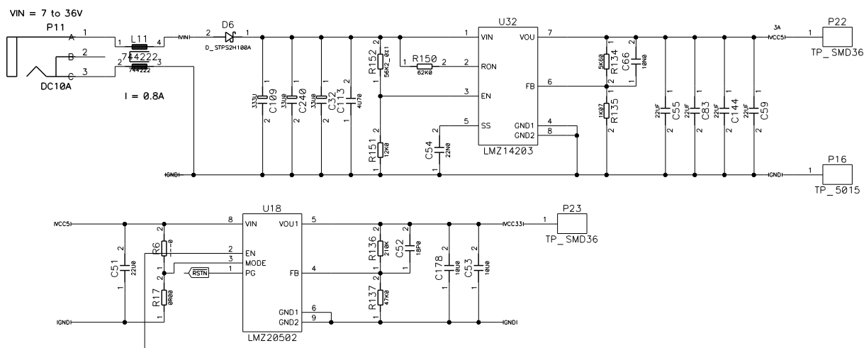
Obr. 2.13 Časť napájania vývojovej dosky
