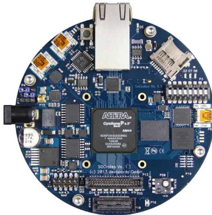
Obr. 2.1 Vývojová doska Socrates na báze FPGA
