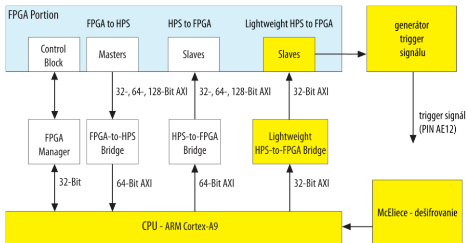
Obr. 2.17 Generovanie trigger signálu pomocou FPGA oddielu SoC čipu (pôvodný spôsob)
