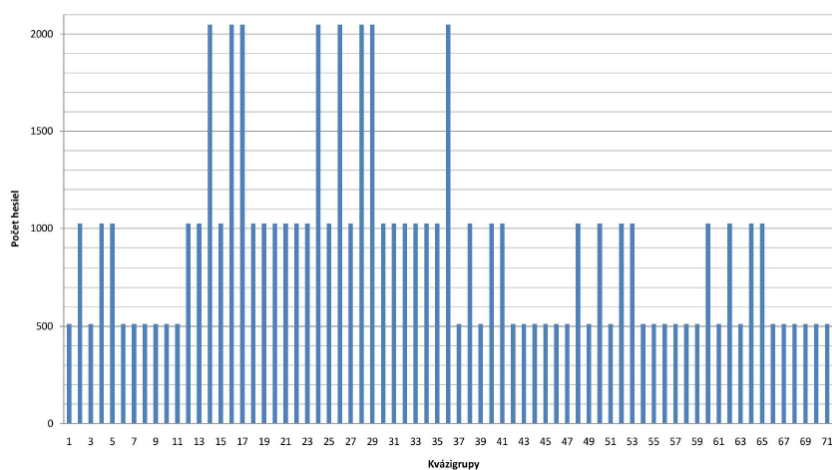
Obr. 4.2 Rozloženie početnosti hesiel pre kvázigrupy rádu 4
