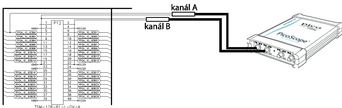
Obr. 2.12 Naznačenie meracích bodov v schéme (konektor P12)
