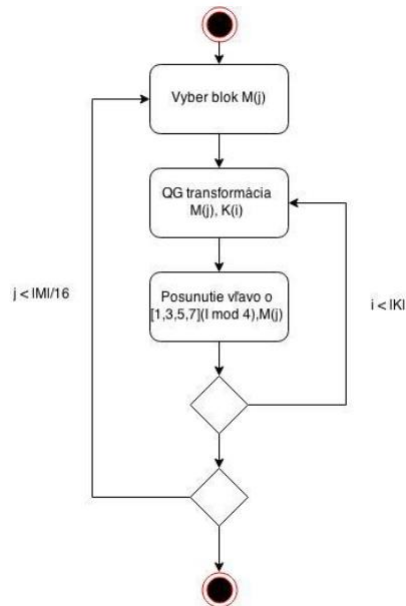
Obr. 4.4 Schéma činnosti kvázigrupovej blokovej šifry
