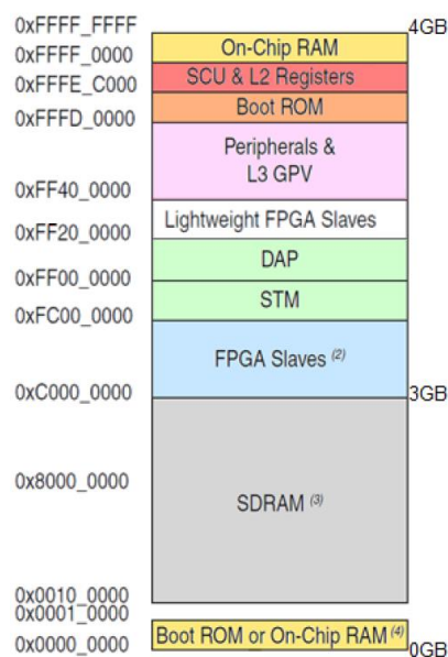
Obr. 2.6 Adresný priestor ARM procesora v SoC systéme
