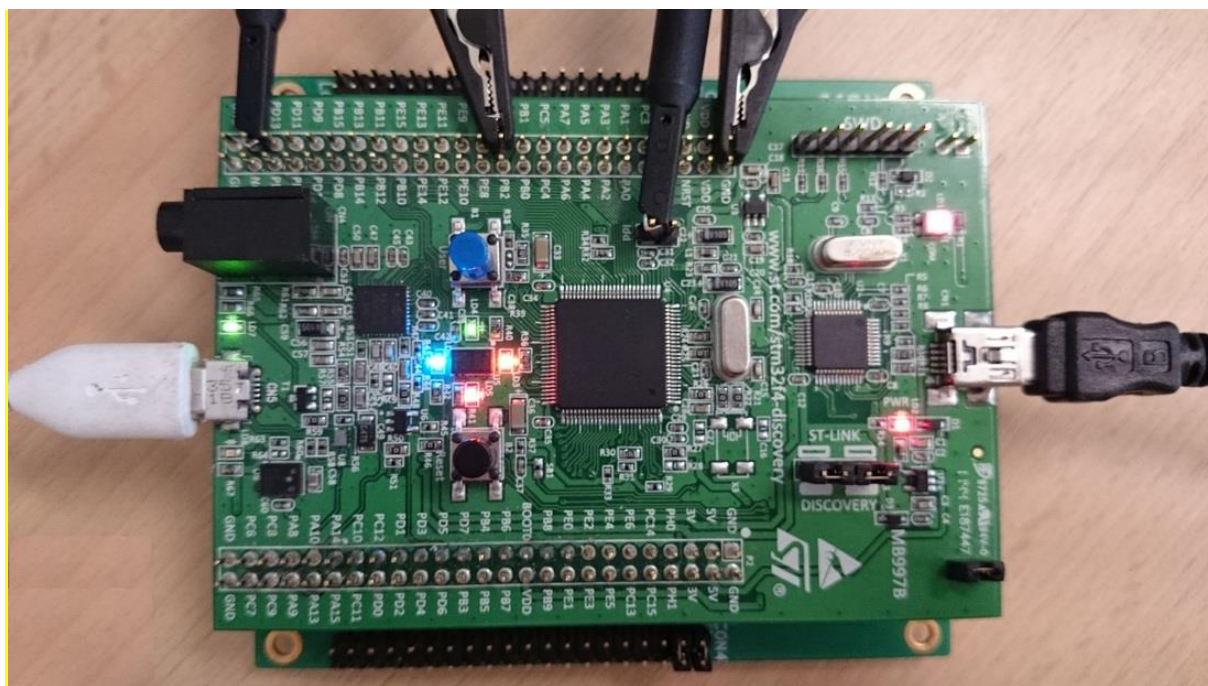
Obr 3.1 Karta STM32F4 s mikroprocesorom STM32F407VGT s rozsvietenými LED diódami, pripojenými sondami na meranie napätia a pripojenými USB káblami zabezpečujúcimi napájanie (čierne miniUSB) a I/O komunikáciu s PC (biele mikroUSB).
