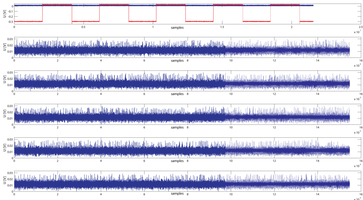
Obr. 2.14 Záznam z merania piatich vektorov spotreby spolu s trigger signálom
