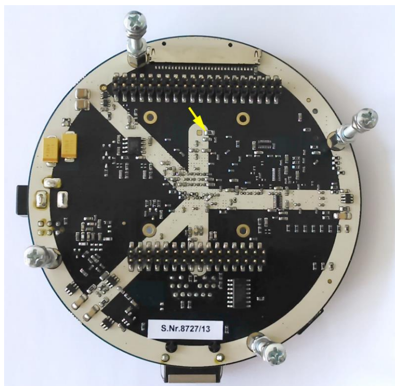
Obr. 2.16 Poloha výhodnejšieho meracieho bodu na meracej doske Socrates
