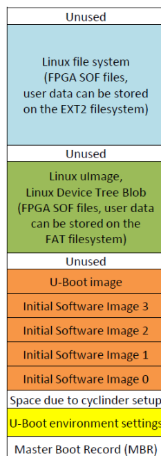
Obr. 2.7 Rozloženie diskových partícií na SD karte
