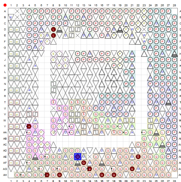
Obr. 2.11 Priradenie umiestnenie vývodu AE12 na entitu trigger_PIO v aplikácii PinPlanner (QUARTUS)
