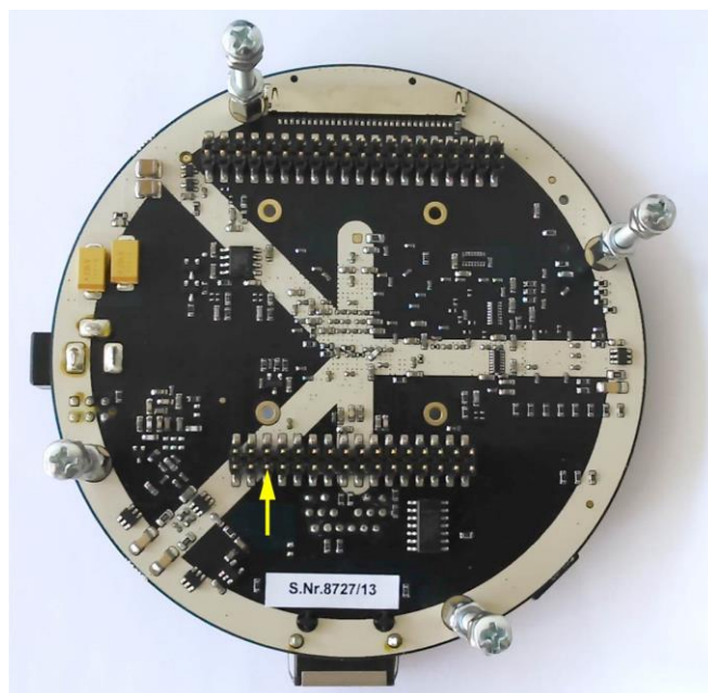
Obr. 2.9 Umiestnenie trigger signálu na konektore P12 (spodná strana dosky)
