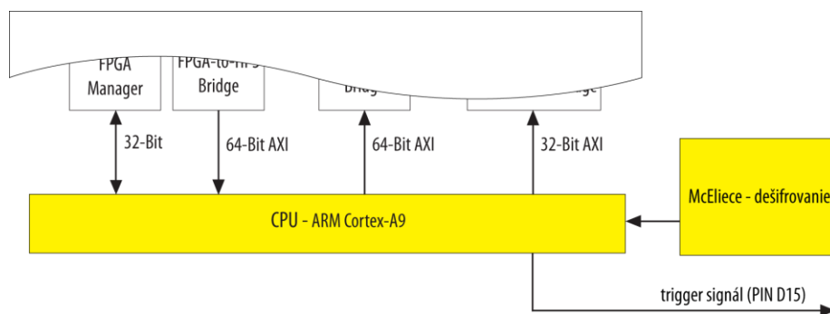
Obr. 2.18 Generovanie trigger signálu pomocou CPU v SoC čipe (nový spôsob)
