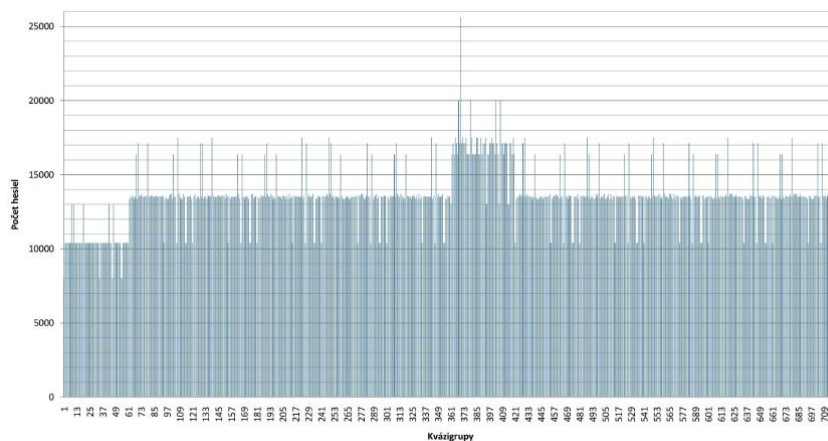
Obr. 4.3 Rozloženie početnosti hesiel pre kvázigrupy rádu 5
