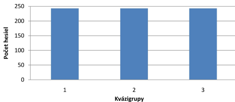
Obr. 4.1 Rozloženie početnosti hesiel pre kvázigrupy rádu 3
